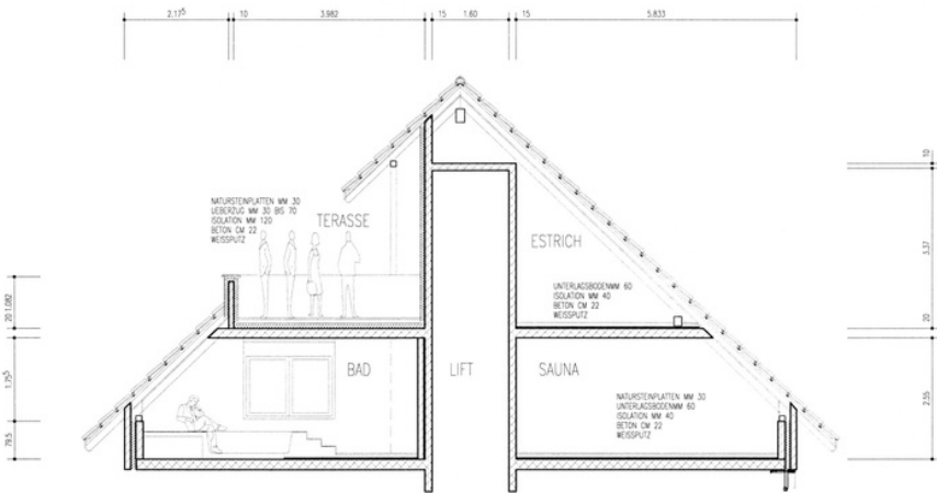
SCHNITT TERASSE
